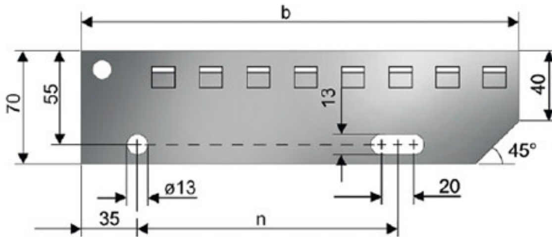
Befestigungssteitenplatte nach DIN 24 531-1
